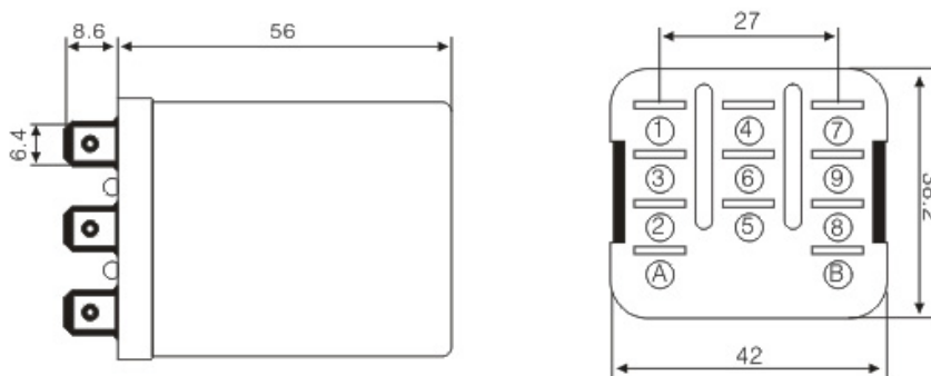
小基座尺寸图
