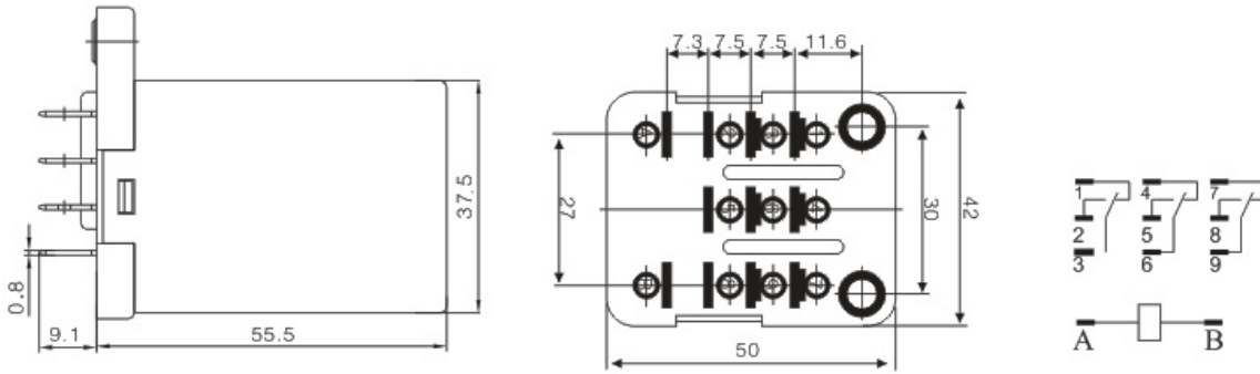
小基座尺寸图
