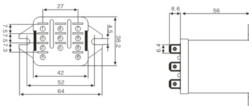
顶部(B)型法兰式尺寸图
