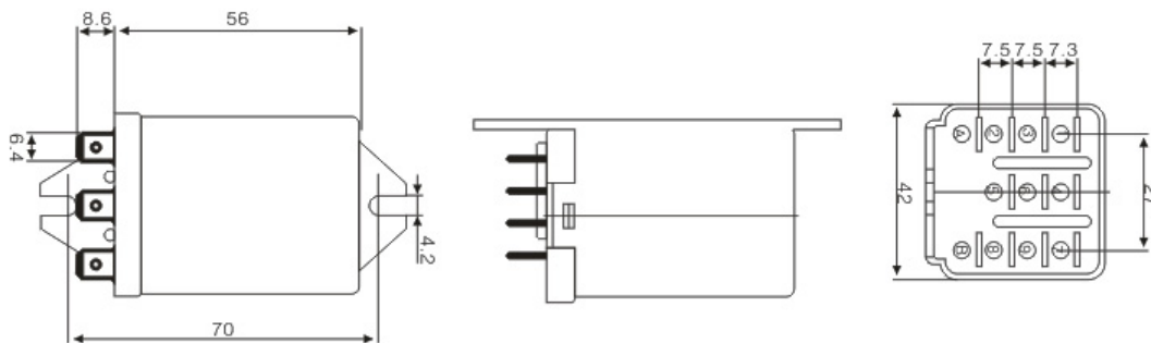
顶部(B)型法兰式尺寸图
